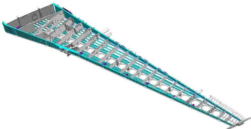
Рисунок 2 - Кессон ОЧК
